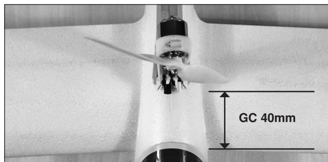
Poloha těžiště je 40 mm při vysunuté pohonné jednotce.
