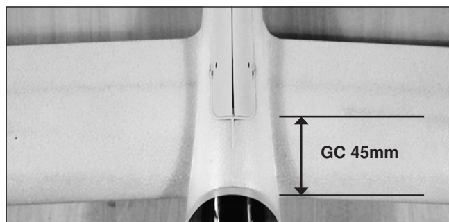
Poloha těžiště je 45 mm při zasunuté pohonné jednotce.
