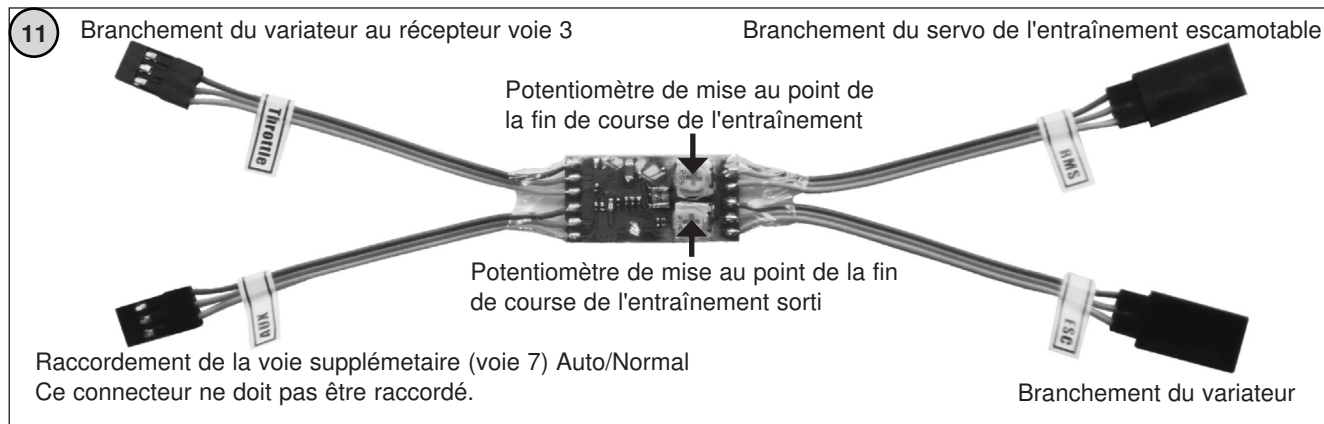
Fig. 11 – 1.1 Module de mixage de l'entraînement escamotable:
