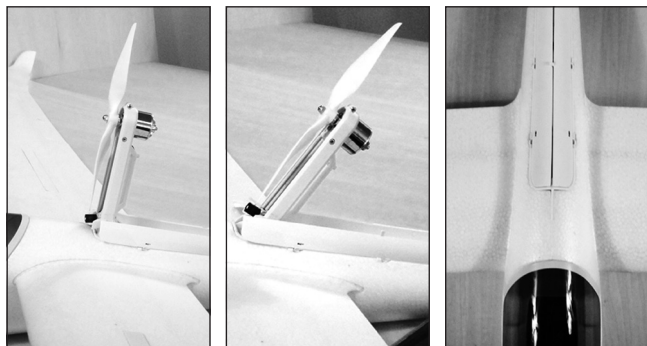
Figura 11 – 1.1 Modulo Mixer per la pinna retrattile:
