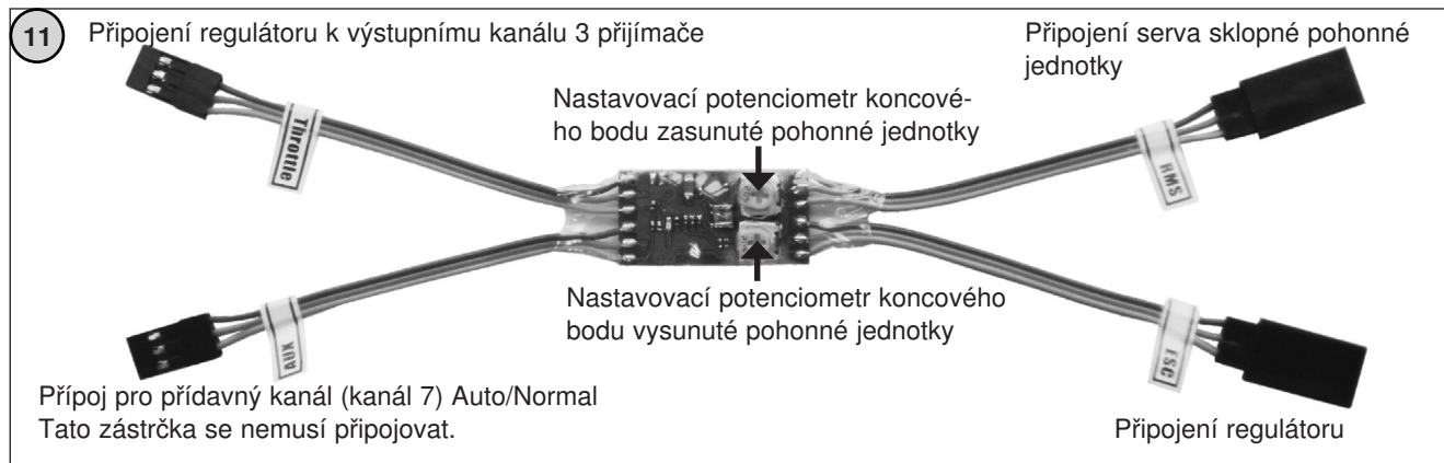
Obr. 11 – 1.1 Modul mixéru pro sklopnou pohonnou jednotku:
